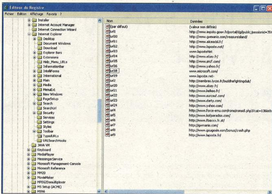
Dans la clé « ...typedURLs », on retrouve l'historique d'Internet Explorer.
